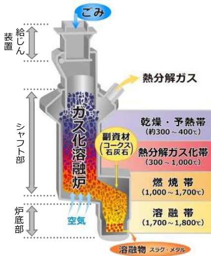
図（シャフト炉式ガス化溶融炉模式）
