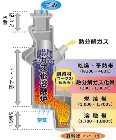
図（シャフト炉式ガス化溶融炉模式）
